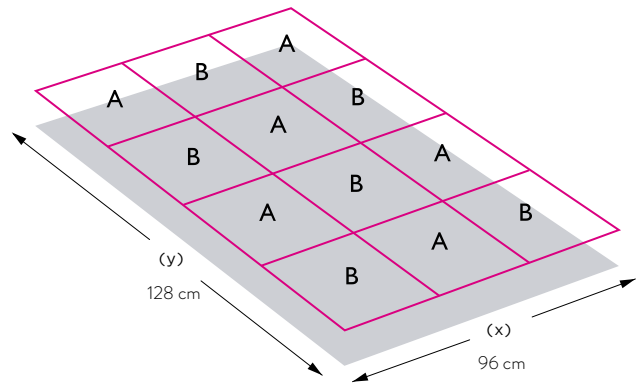
Ejemplo de emplatado de modelo con 2 módulos: Mounting example of a design made from 2 modules:
